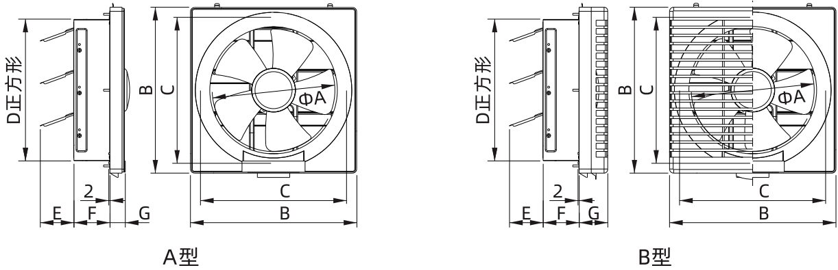
外型及部件尺寸
