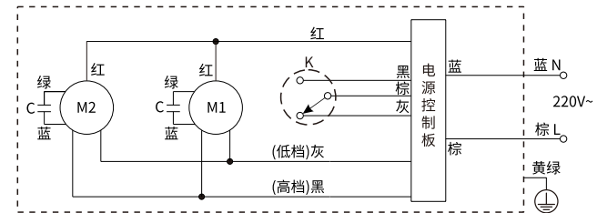
原理图适用 FM5509L ,FM5512L
