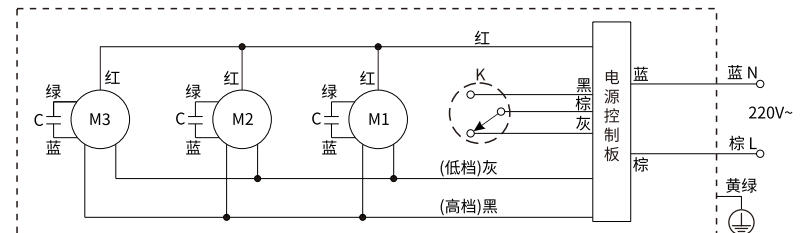
原理图适用 FM5515L ,FM5518L ,FM5520L
